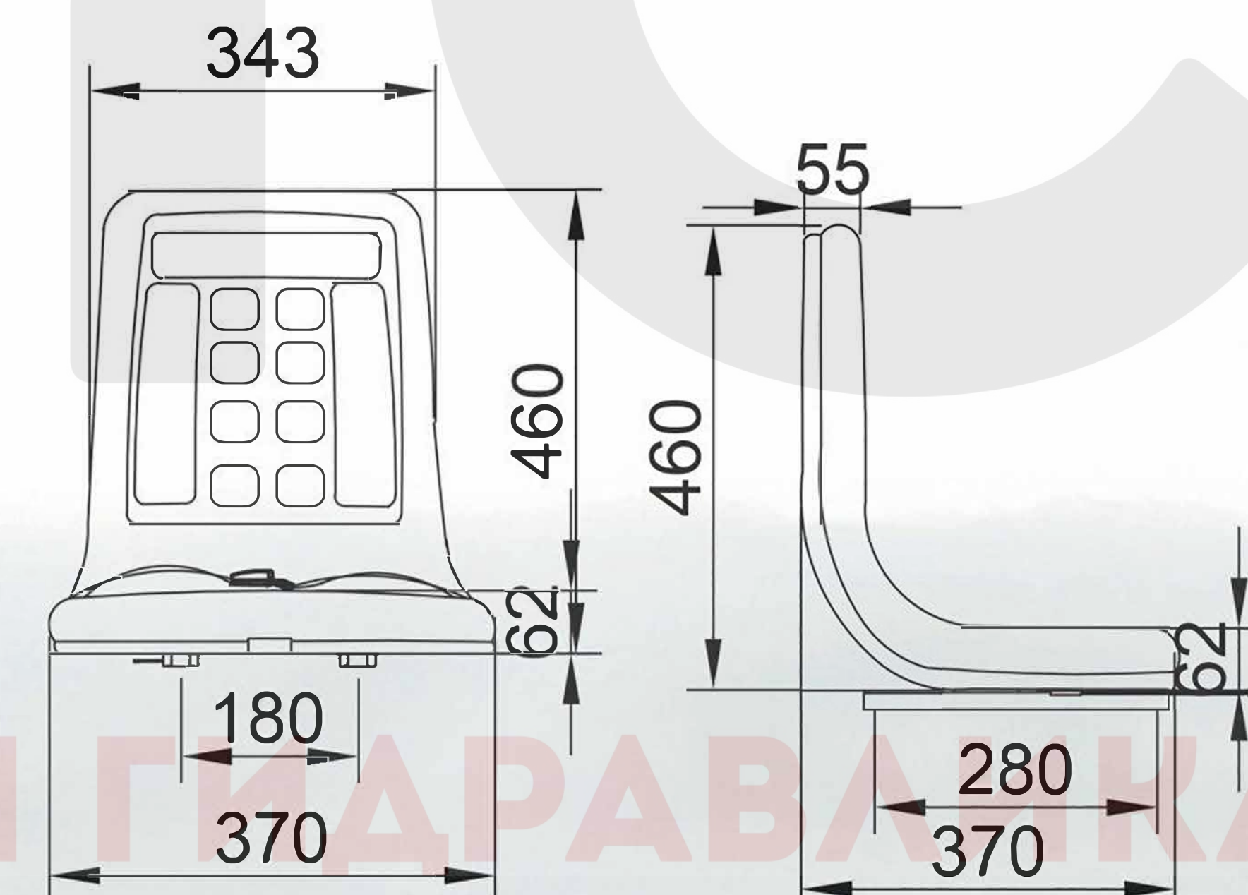
型号:FD-808-3 MODEL:FD-808-3
