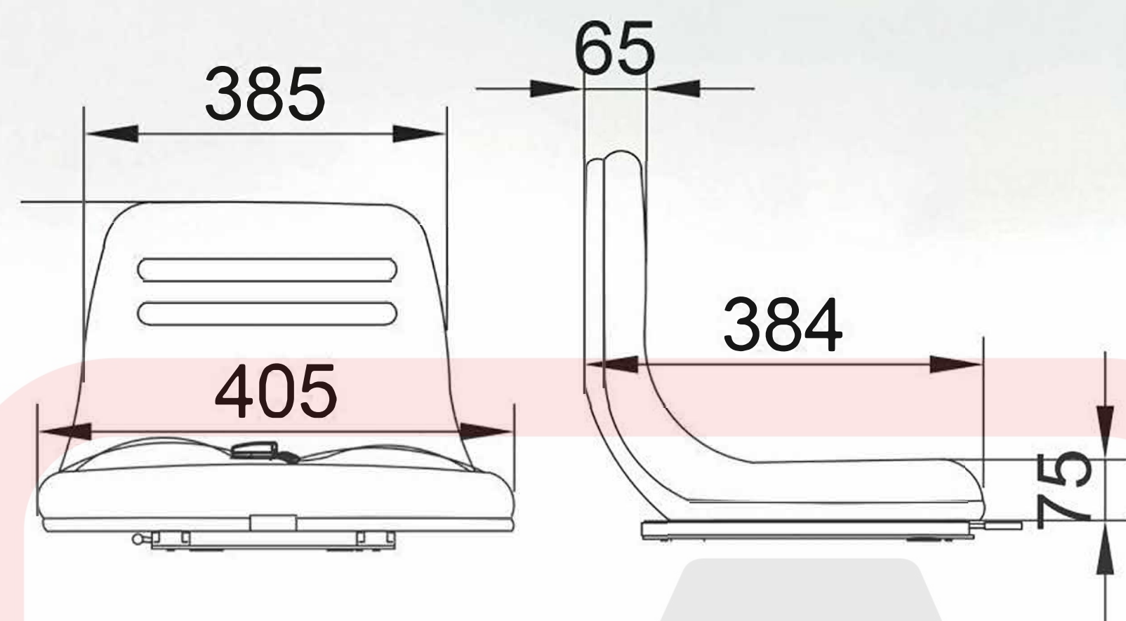
型号:FD-808-3 MODEL:FD-808-3
