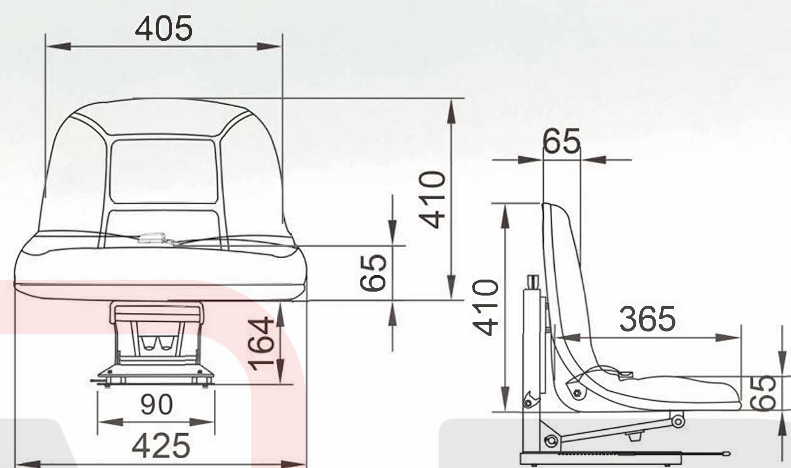
型号:FD-858-1 MODEL:FD-858-1
