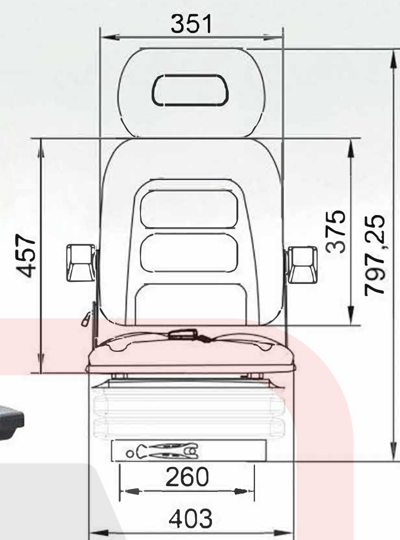
型号:FD-801 MODEL:FD-801
